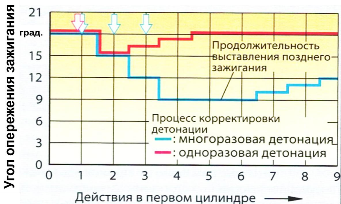
Рисунок 4.18 – Регулирование момента зажигания во время детонации
