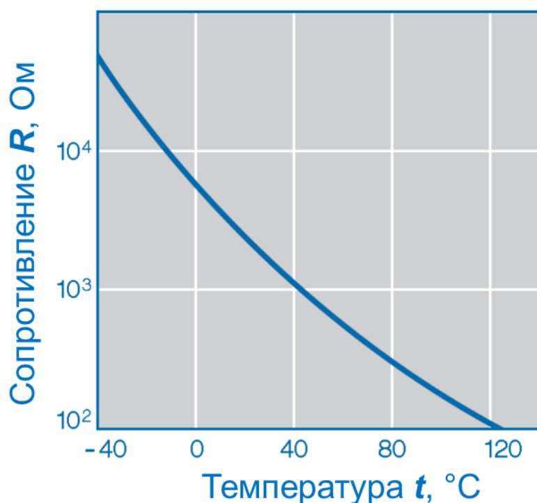
Рисунок 4.23 – Выходная характеристика датчика температуры двигателя
