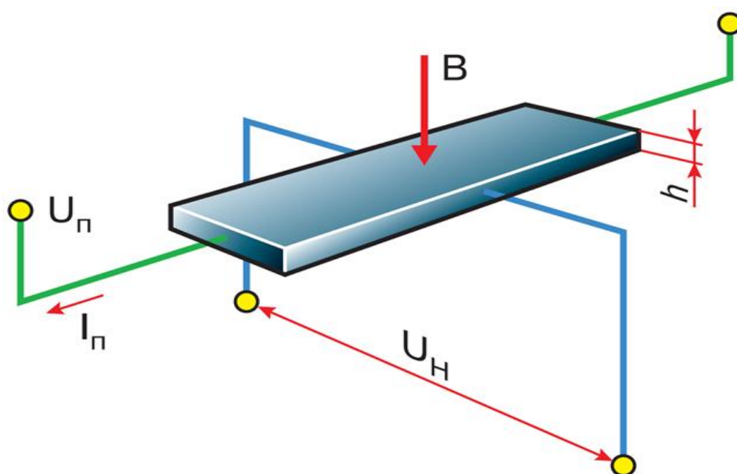
Рисунок 4.3 – Эффект Холла
