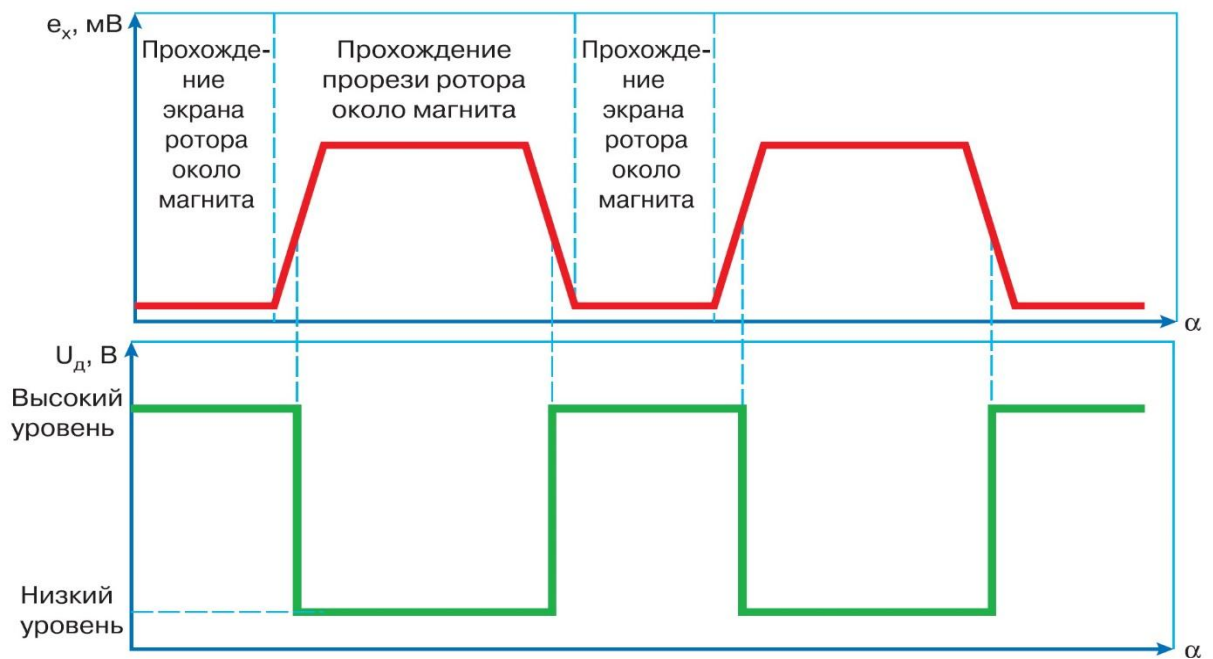
Рисунок 4.5 – Выходной сигнал датчика Холла
