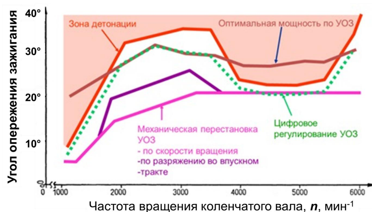
Рисунок 4.12 – Оптимальное изменение угла опережения зажигания по детонации
