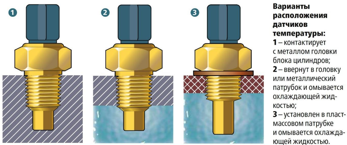
Рисунок 4.24 – Расположение датчиков температуры двигателя
