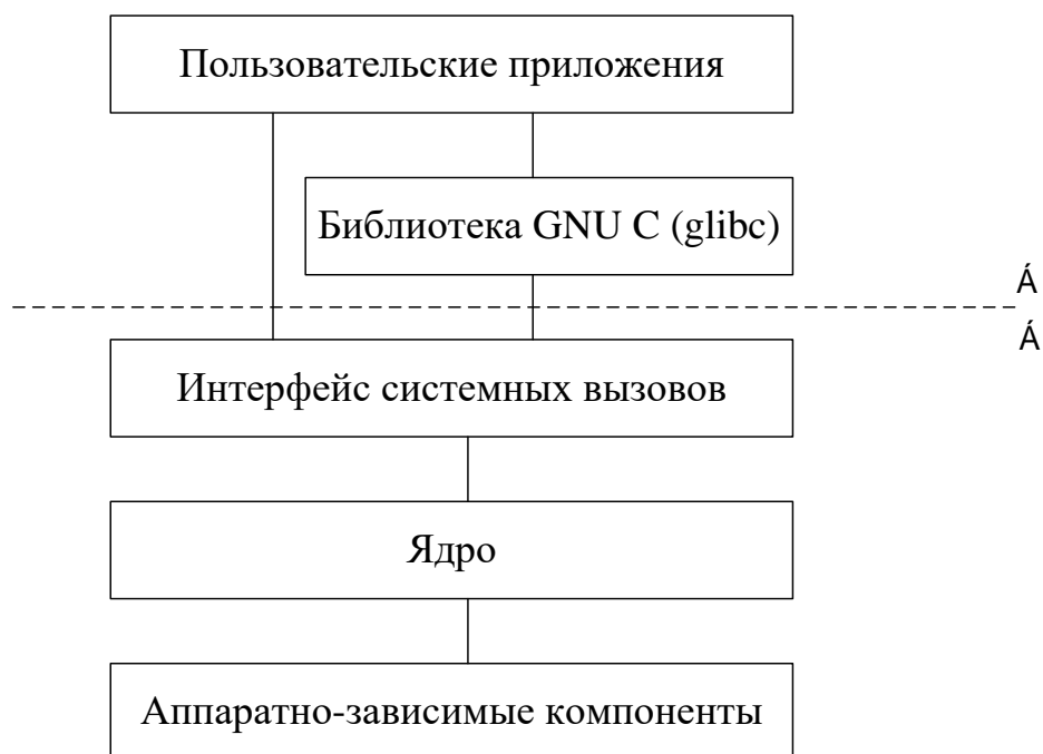
Рисунок 8 – Упрощенная структура GNU Linux
