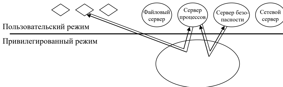
Рисунок 4 – Сема организации системного вызова в микроядерной ОС
