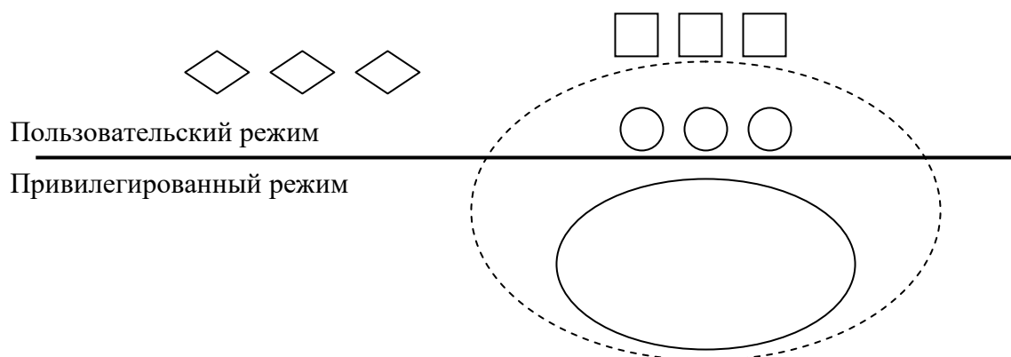
Рисунок 3 – Микроядерная архитектура
