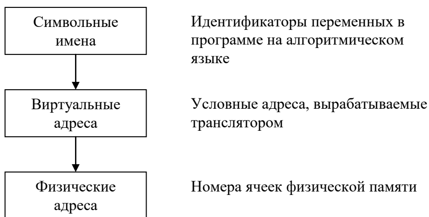
Рисунок 22 – Типы адресов
