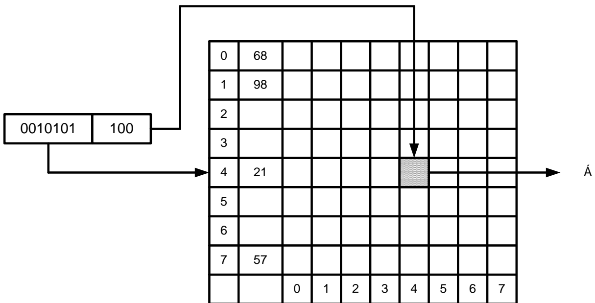
Рисунок 32- Схема работы ассоциативной кэш-памяти
