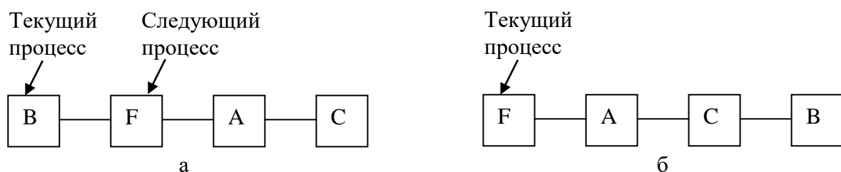
Рисунок 18 – Циклическое планирование
