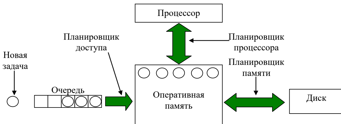
Рисунок 17 – Трехуровневое планирование
