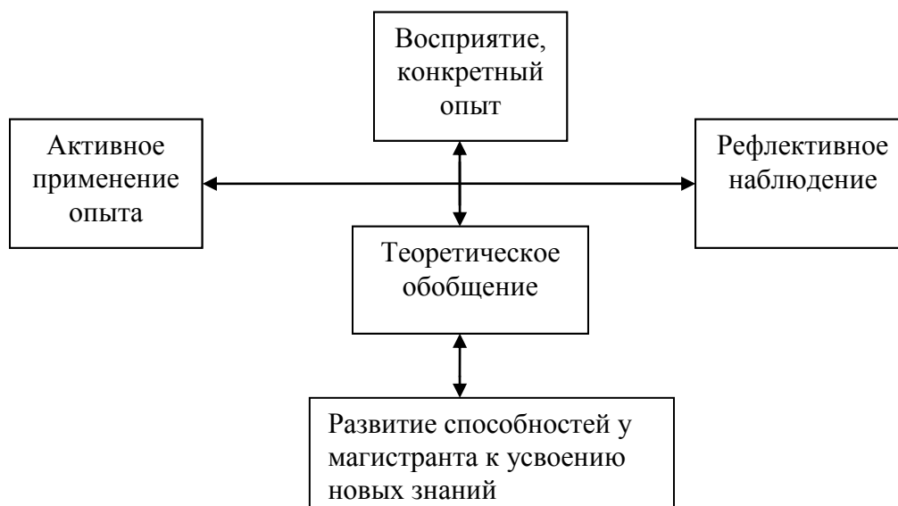
Рисунок 2 – Модель обучения
