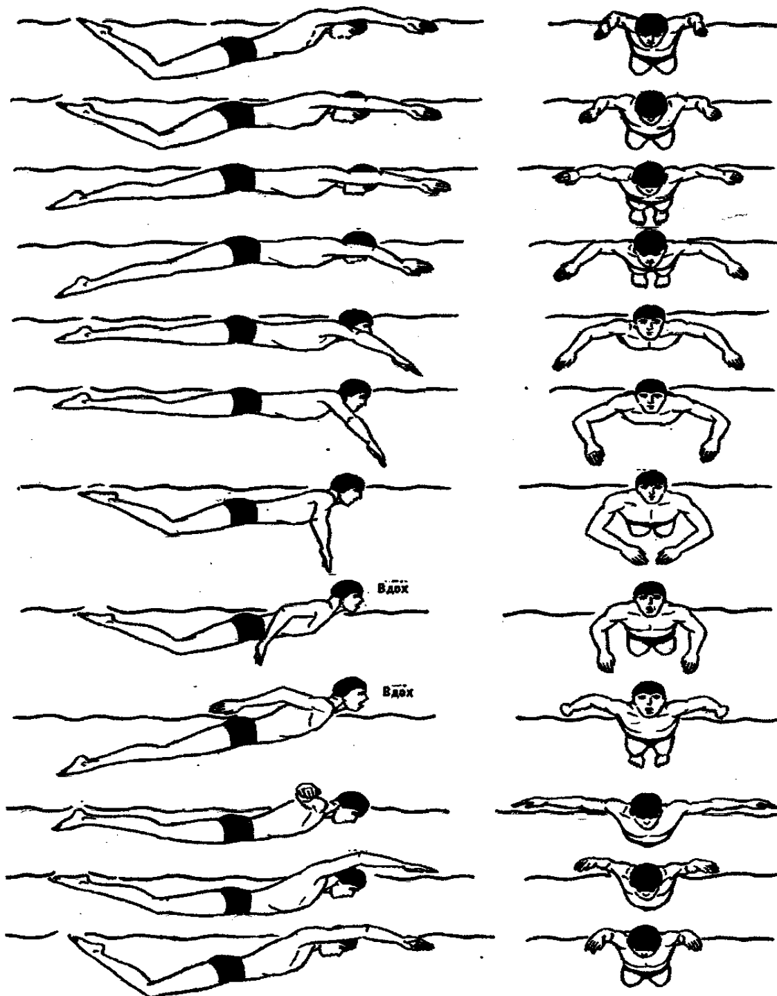
Рисунок 4 – Баттерфляй
