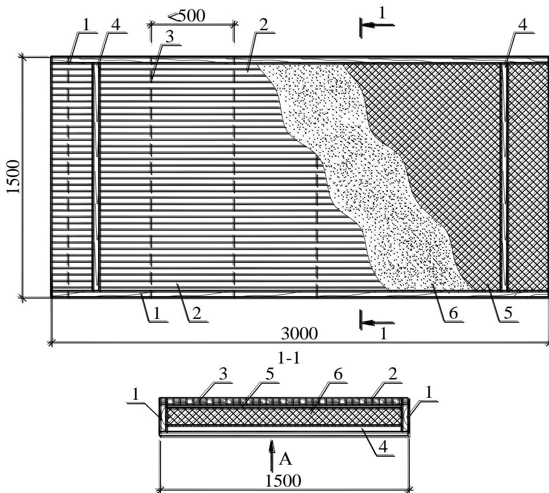
Рис. 1. Унифицированы элемент П-образного сечения:
