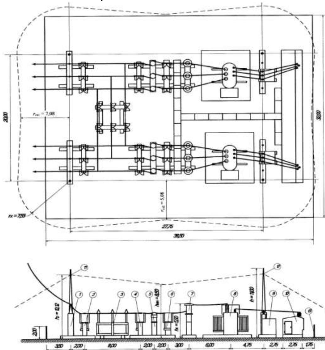
Рисунок 1 - План и зона молниезащиты
