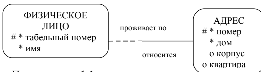
Рисунок 28 — Пример связи 1:1
