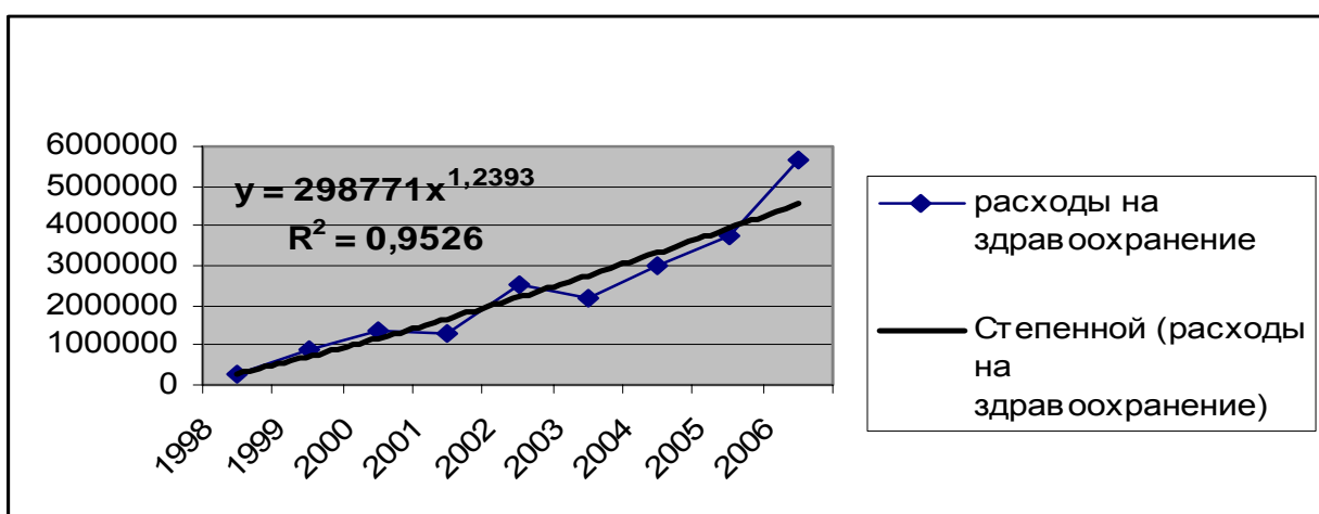
Рисунок 4 – Степенной тренд
