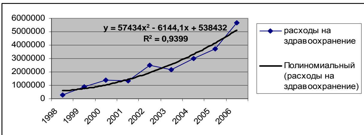
Рисунок 3 – Полиномиальный тренд
