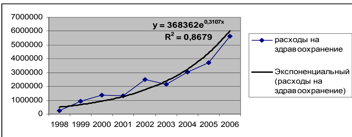
Рисунок 5 – Экспоненциальный тренд
