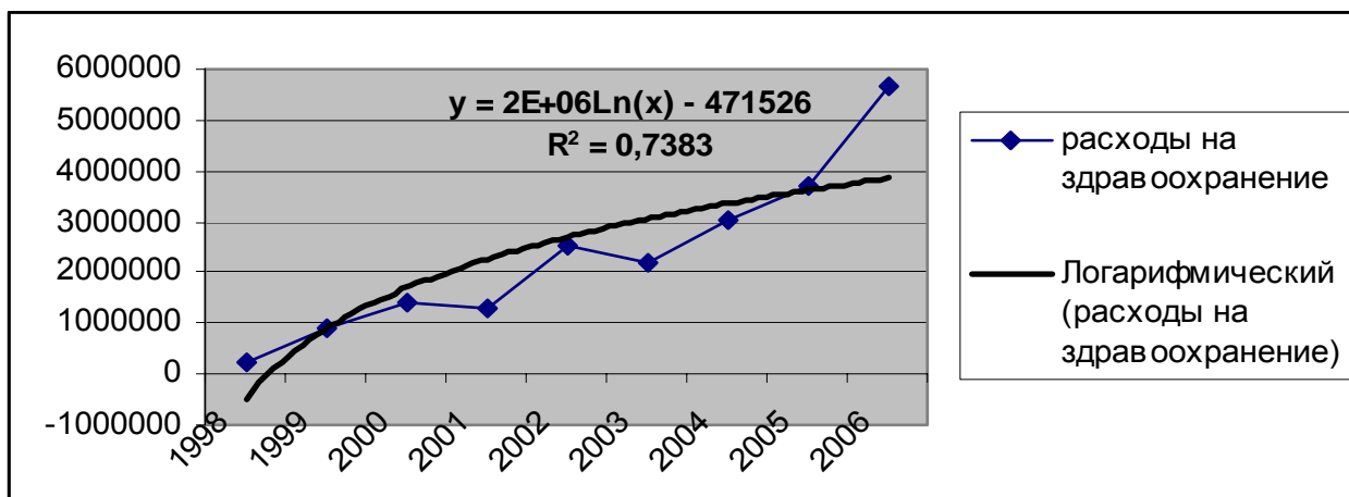
Рисунок 2 – Логарифмический тренд
