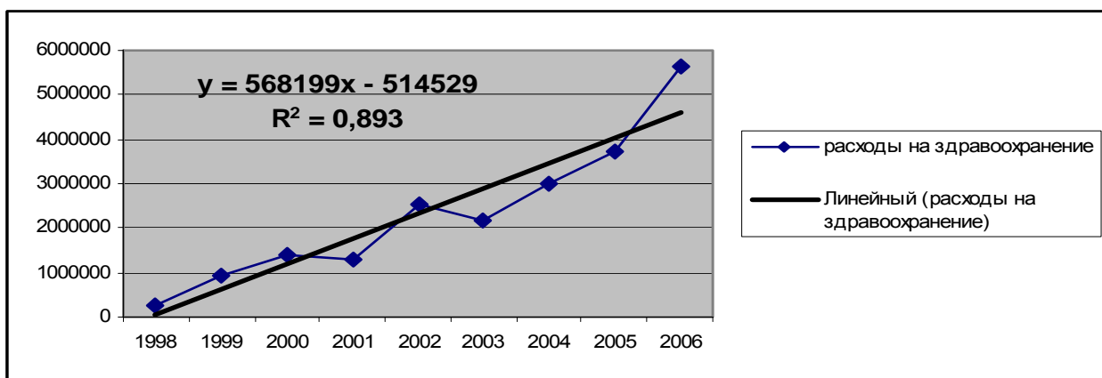
Рисунок 1 – Линейный тренд
